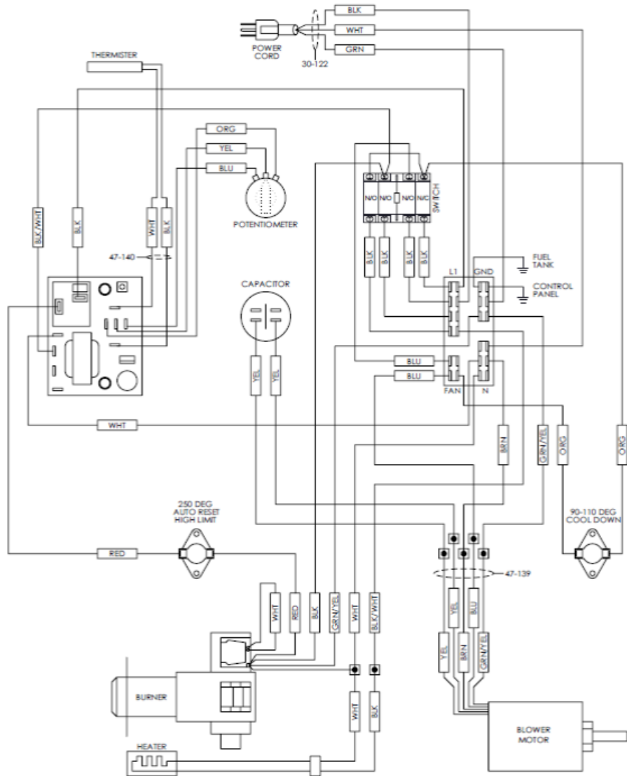
WIRING SCHEMATIC - DRAGON 3600
