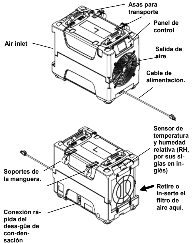
Imagen A: Identificación de las piezas
